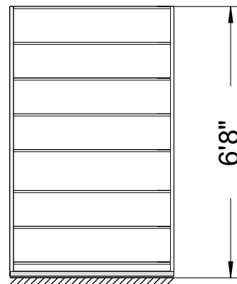
48x24 Elevation
