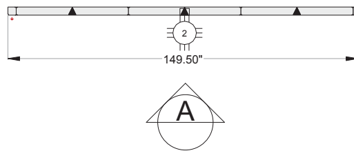
Elevation A
