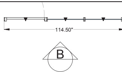
Elevation B
