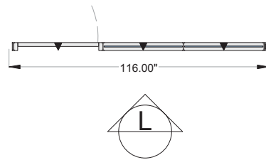
Elevation L
