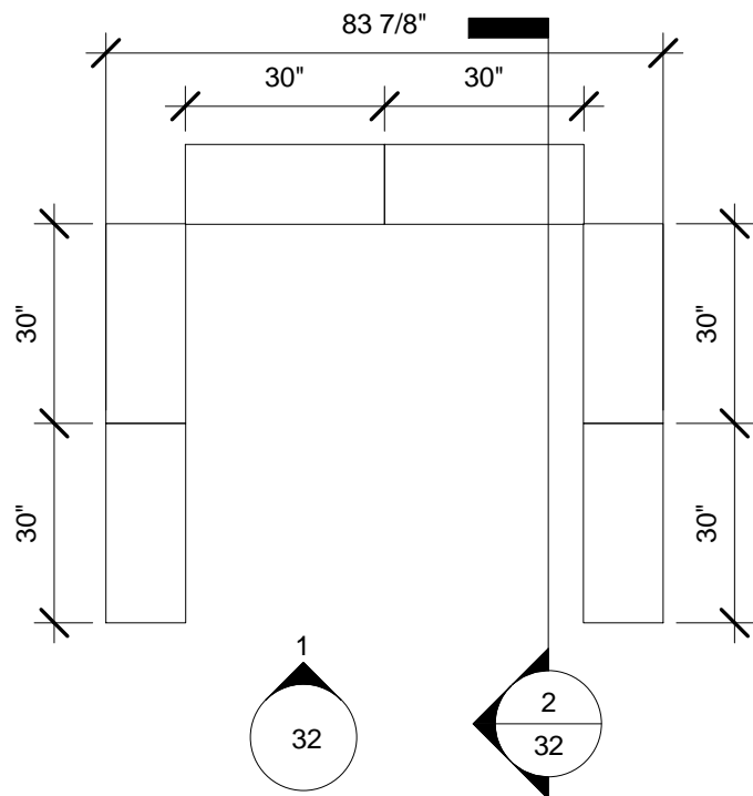
① 7' - Option 7 3/8" = 1'-0"
