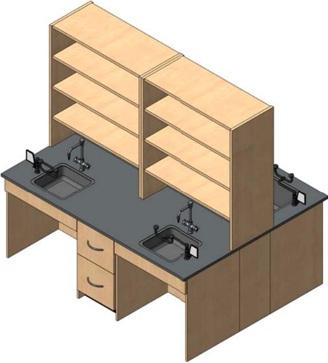
② 7' - Option 2
