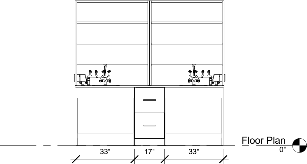
2 7' - Option 2-A 3/8" = 1'-0"
